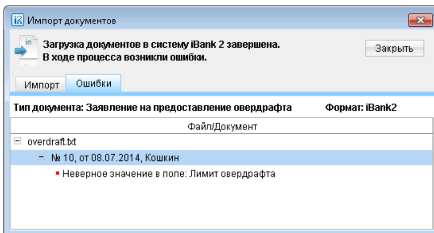
Рис. 3.4. Окно Ошибка
